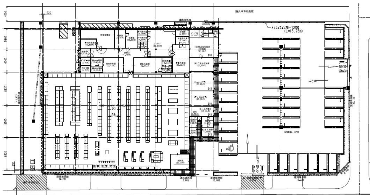
施設全体平面図
